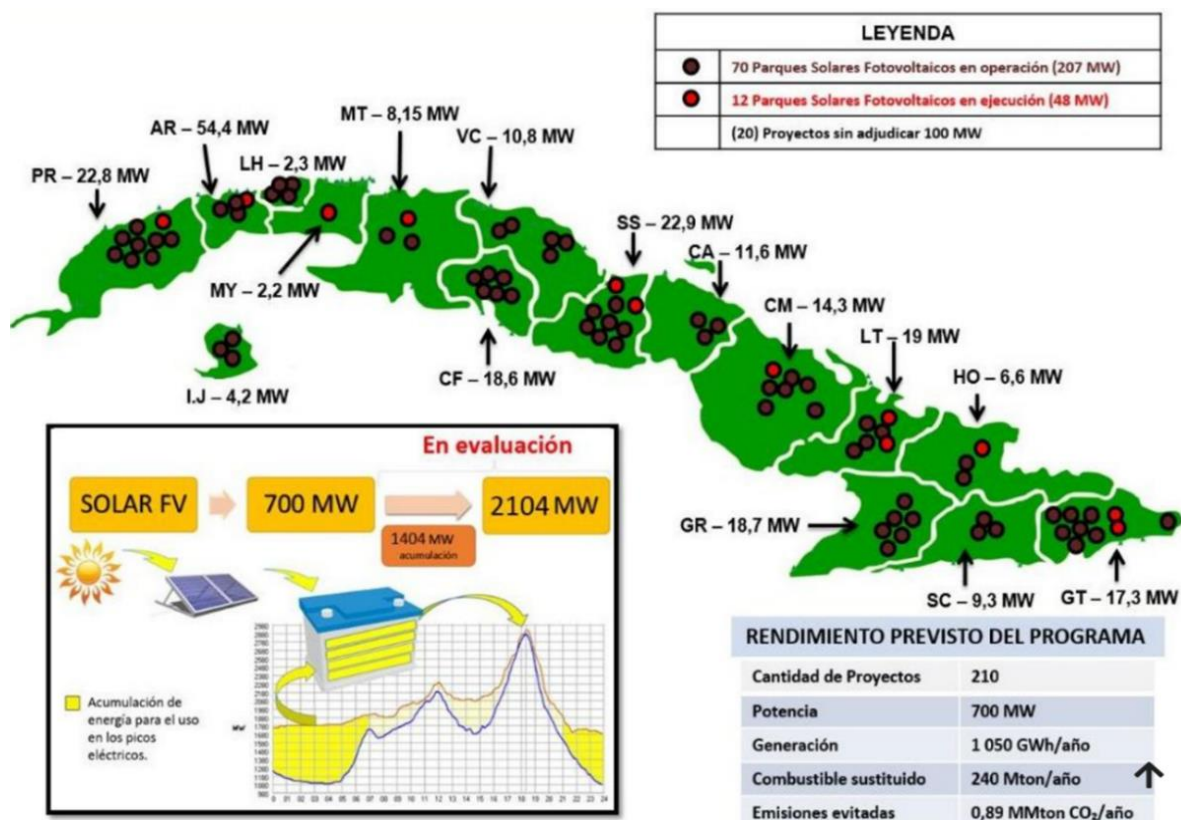
Figura 12. Programa Solar Fotovoltaico Fuente: MINEM, 2025.
