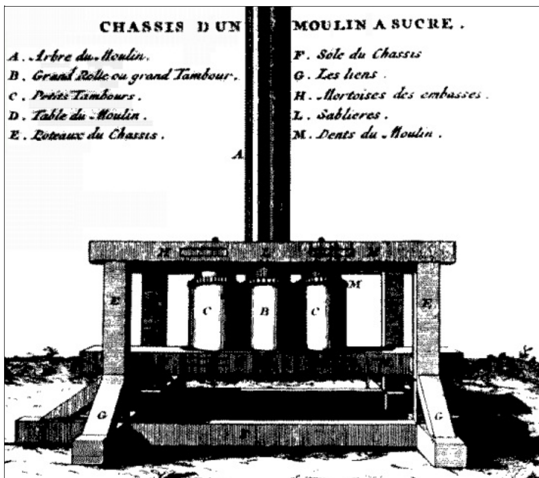
TÍPICO TRAPICHE VERTICAL DEL SIGLO XVIII
